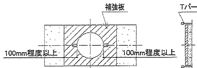
図3. ライン・長尺タイプ（設備ゾーン）天井材補強の例
