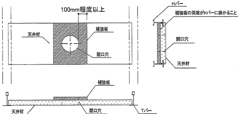
図4. ラインタイプ、長尺ラインタイプ天井材補強の例
