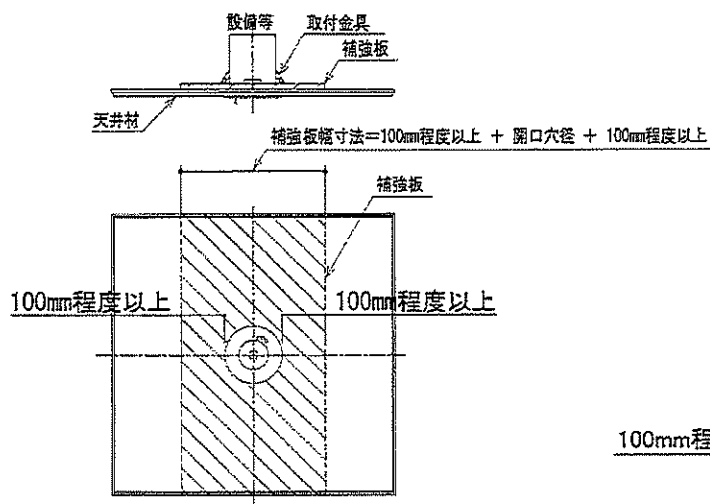
図2. グリッドタイプ天井材補強の例
