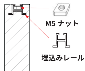
断面
