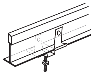
回転クリップをTバーに取付けた状態
