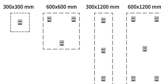
パネルサイズによる専用グリップ数（参考）
