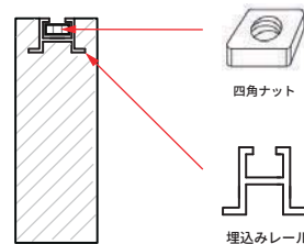
断面図 a) - a)
