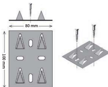
ビス止め箇所はボードの下地に合わせてください。
